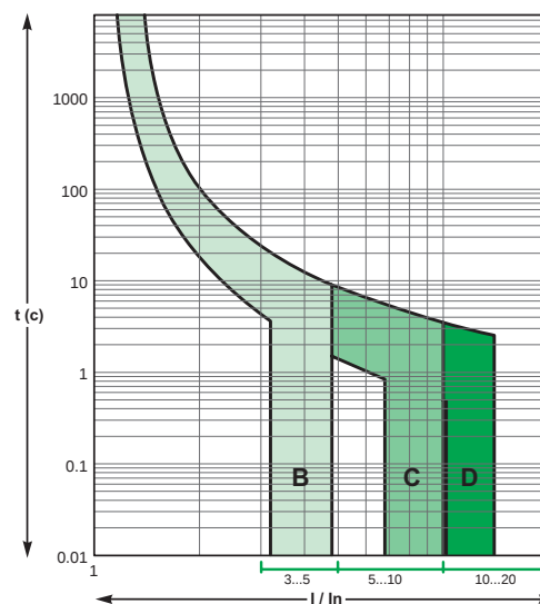
Кривые отключения
