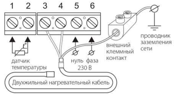
Схема подключения нагревательного кабеля «ONEKEYELECTRO» ОКЕ
