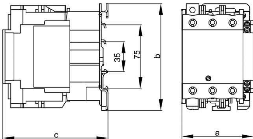
Рисунок 4 – Габаритные размеры контакторов КМИ-A-46512 – КМИ-A-49512
