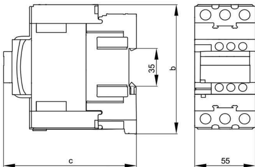
Рисунок 3 – Габаритные размеры контакторов КМИ-А-34012, КМИ-А-35012
