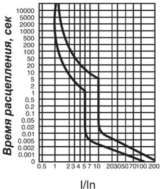
Рис. 2. Кривая отключения C
