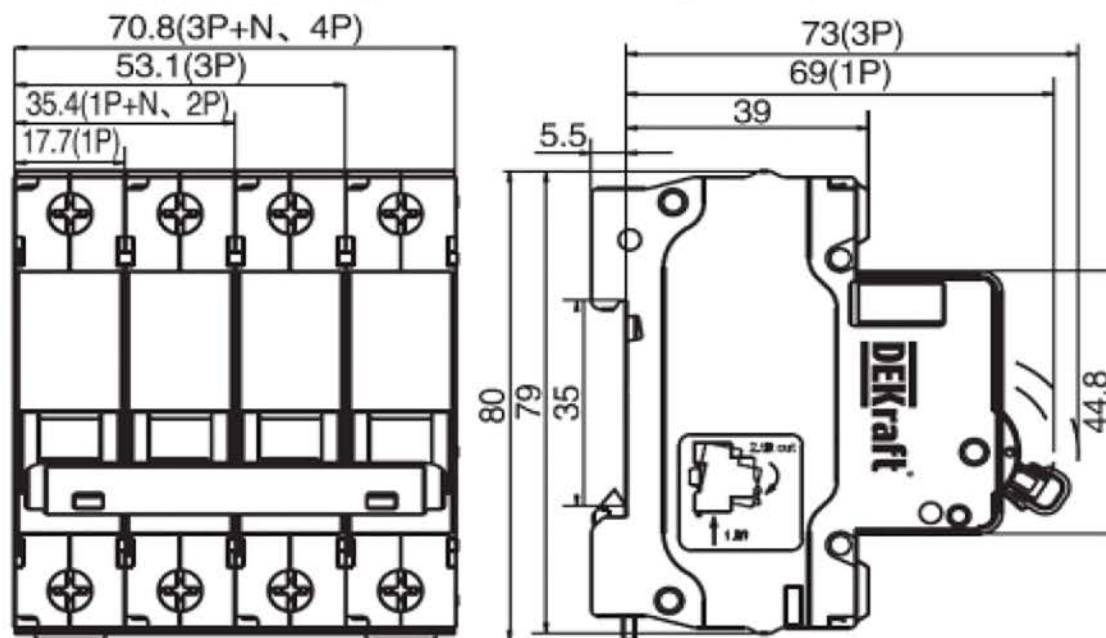
Рис. 4. Габаритные размеры аппаратов серии BA-101, мм
