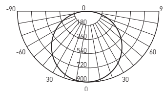
PTR 1935 35w
