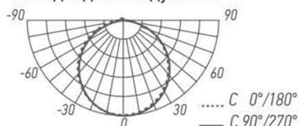
Светодиодный модуль. Тип F
