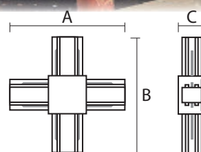
Коннектор X-образный
