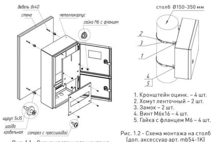
Рис. 1.1 - Схема настенного монтажа
