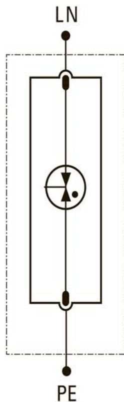
Рисунок 5 – Схема подключения УЗИП Т1 1Р ЕКФ
