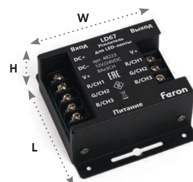
Усилитель для светодиодной ленты, RGB
