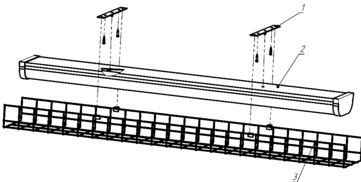
Рисунок 1. Схема монтажа защитной решётки
