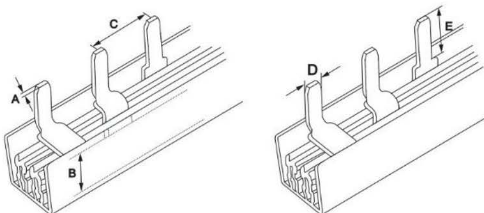
Рисунок 6 – Шина типа PIN 2P 63, 100 А
