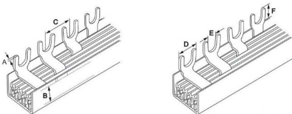
Рисунок 3 – Шина типа FORK 3P 63, 100 А
