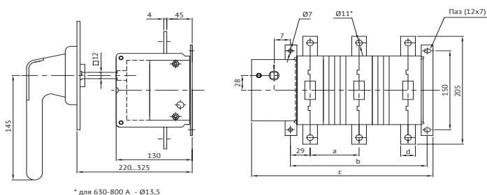
OptiSwitch DI-3-(400-800A)
