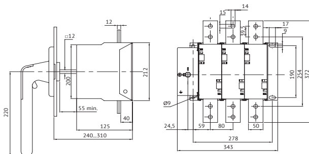
OptiSwitch DI-4-(1000-1250A)
