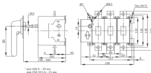
OptiSwitch DI-2-(200-315A)
