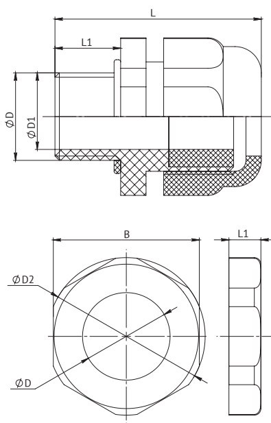
Сальники РГ
