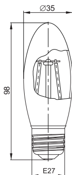
Рисунок 3 – Лампа LED-C35 серия 360° 5 Вт, 7 Вт цоколь E27
