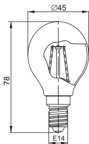
Рисунок 4 – Лампа LED-G45 серия 360° 5 Вт, 7 Вт цоколь E14
