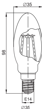
Рисунок 2 – Лампа LED-C35 серия 360° 5 Вт, 7 Вт цоколь E14
