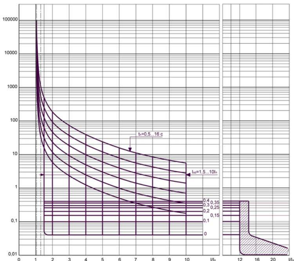
Рисунок 2 - Время-токовая характеристика выключателей
