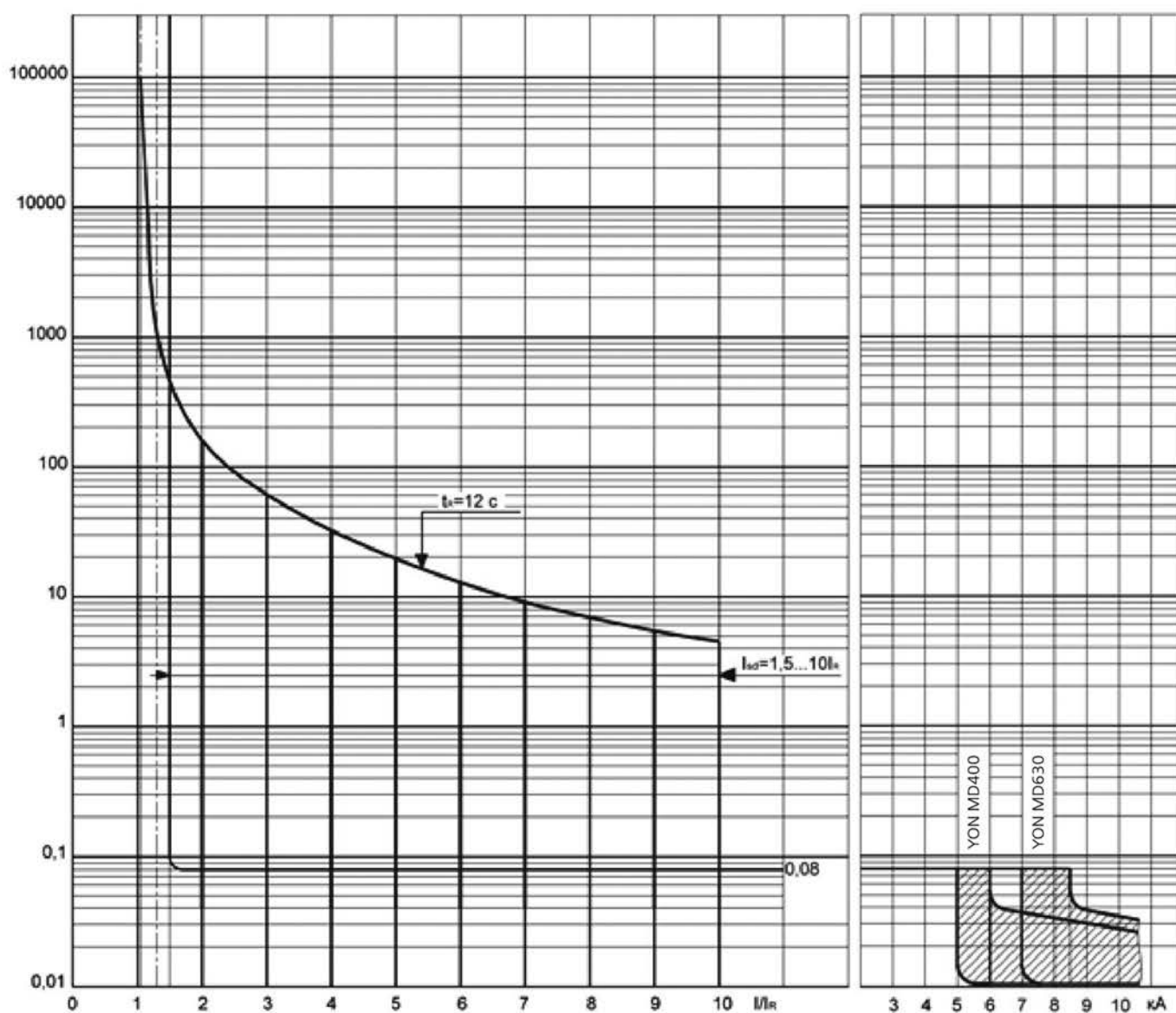
а) – для выключателей с применением расцепителя MR1
