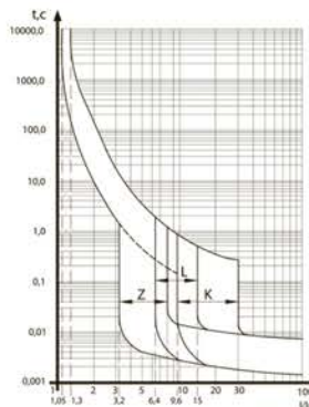
Рисунок Б.8 Защитная характеристика по ГОСТ IEC 60947-2 в цепи постоянного тока при контрольной температуре плюс 45°C.
