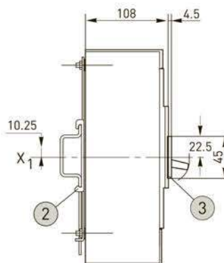
3 Разделительная пластина
