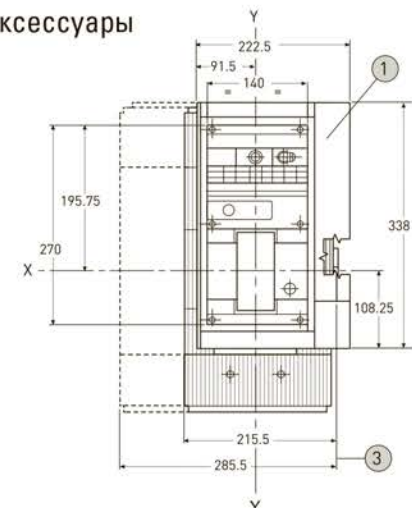
① Передний фланец для двери шкафа (прилагается)
