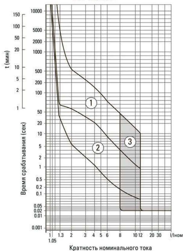
ВА-99/400
