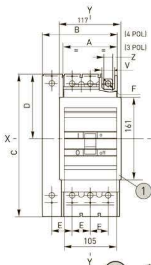
1 Фланец для двери шкафа
