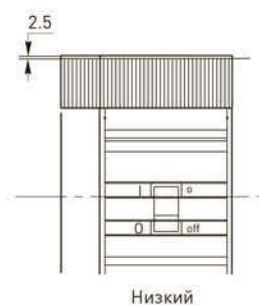
3 Разделительная пластина
