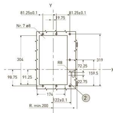
③ Размеры с соединителями
