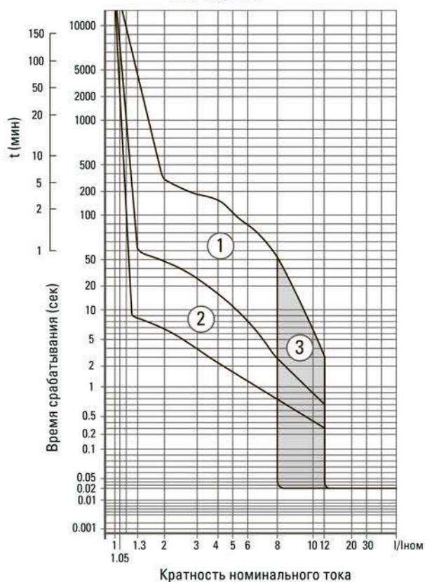
ВА-99/250
