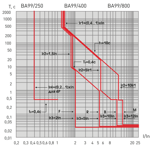
Характеристика расцепления выключателя при включении по I^2t
