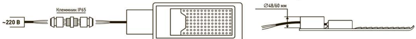
Рис.1. Схема подключения светильника к сети 220В.
