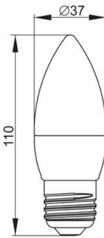
Рисунок 7 – Лампа LED-C35, 7 Вт, 9 Вт, цоколь E27
