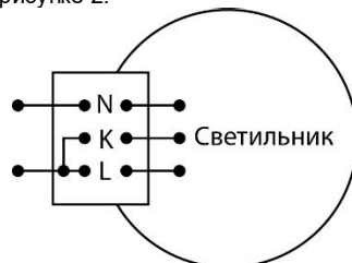
Рис. 2 Схема подключения
