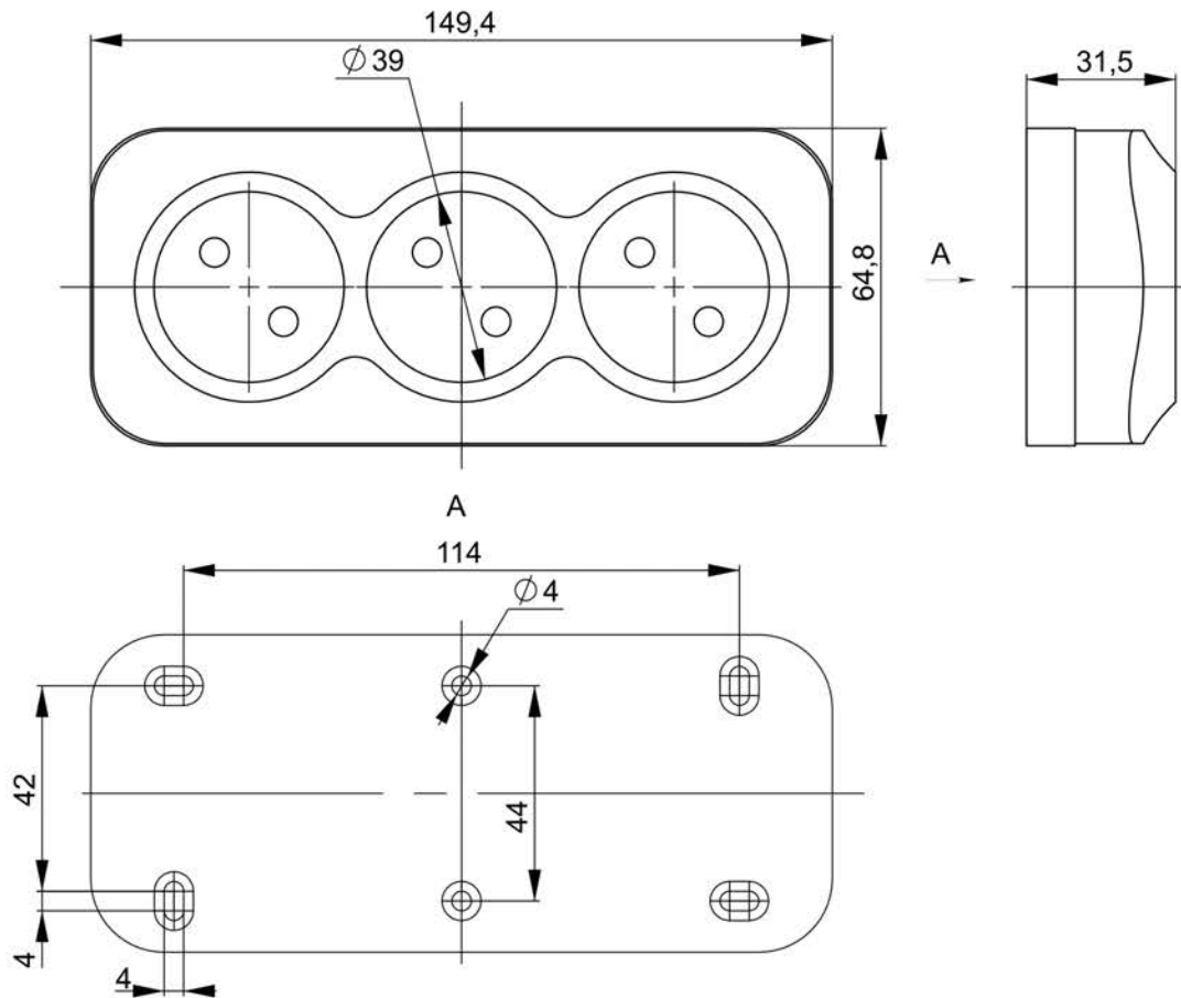
Рисунок 6 – Габаритные и установочные размеры розеток PC23-2
