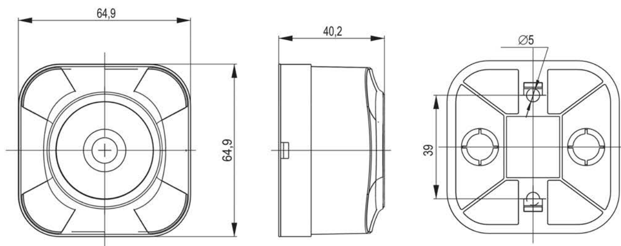
Рисунок 5 – Габаритные и установочные размеры телефонных розеток серии GLORY
