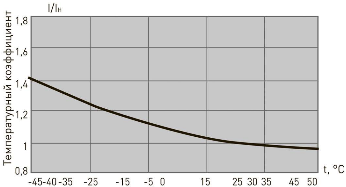
Рис. 2. Температурный коэффициент
