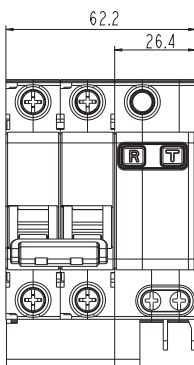
ДИФ-101 2P 32А
