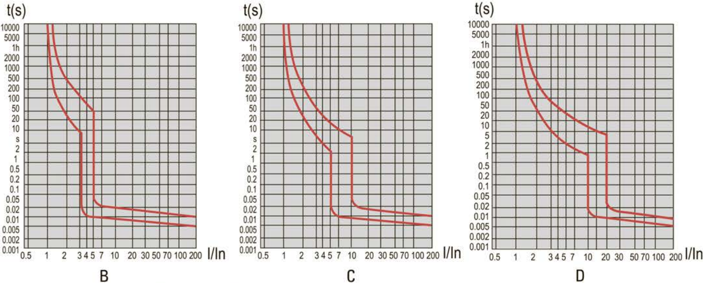
Рис. 1. Время-токовые характеристики
