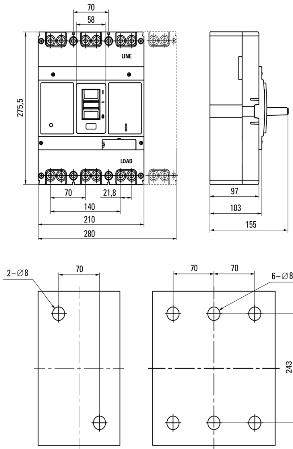
Габаритные размеры ВА-99М 1250 с электронным расцепителем
