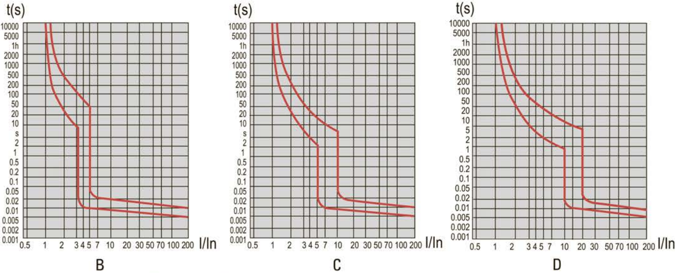
Рис. 1. Время-токовые характеристики
