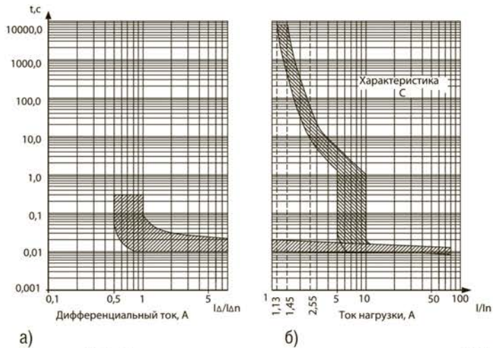
Рисунок Б.1 - Время-токовые характеристики отключения АВДТ
