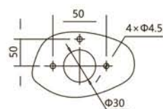
Отверстия в двери шкафа для монтажа выносной рукоятки
