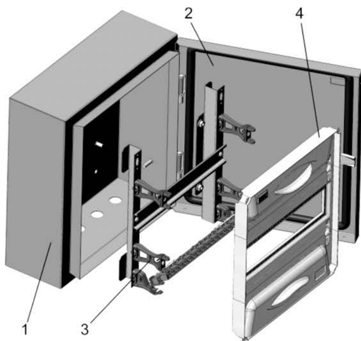
Рисунок 1 – Состав изделия
