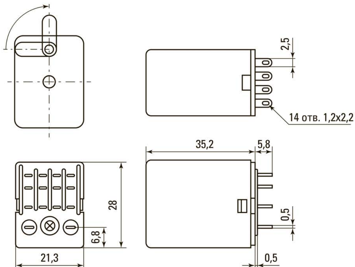
Рис. 4 Габаритные размеры реле промежуточное RPA 22/4 5A EKF AVERES
