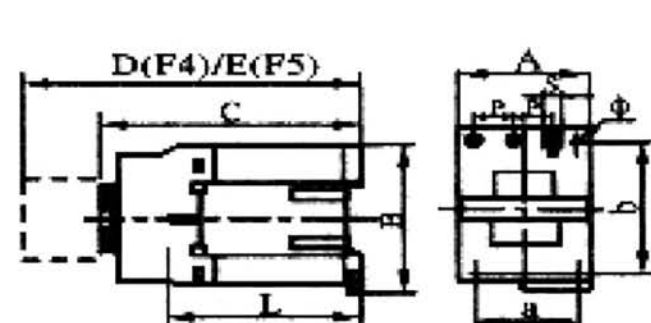
Рисунок 3- Габаритные и установочные размеры контактора NC1-09Z~32Z
