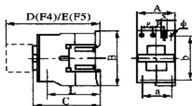
Рисунок 1- Габаритные и установочные размеры контактора NC1-09-32
