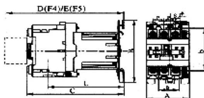
Рисунок 4- Габаритные и установочные размеры контактора NC1-40Z~95Z
