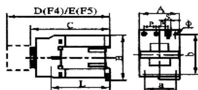
Рисунок 3- Габаритные и установочные размеры контактора NC1-09Z~32Z
