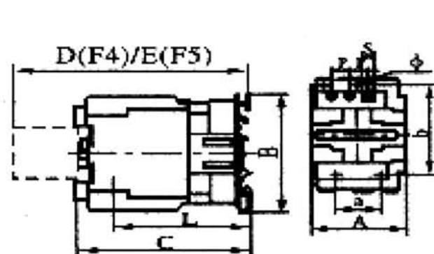
Рисунок 2- Габаритные и установочные размеры контактора NC1 40-95
