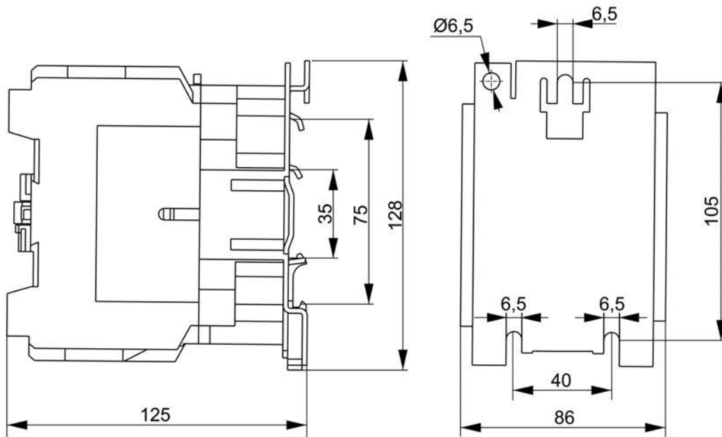
Рисунок 5 – Габаритные и установочные размеры КМИе-48012, КМИе-49512
