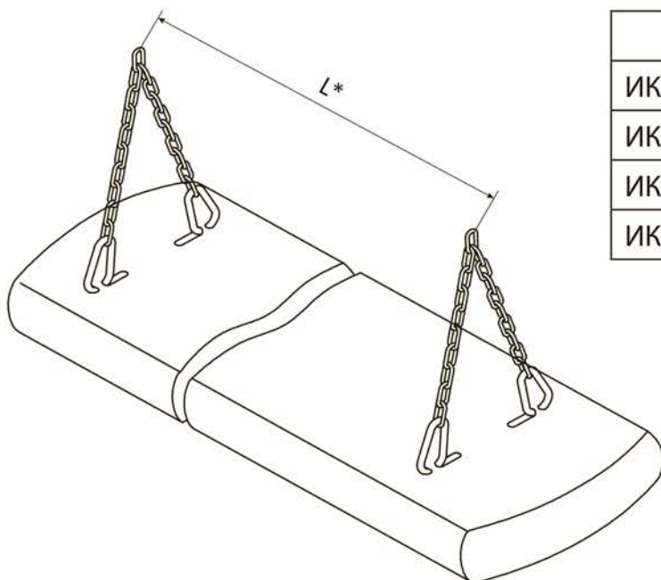
Рисунок 4. Монтаж обогревателей
