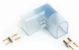
Соединитель угловой для ленты LS720, LS721
