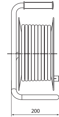
Удлинитель силовой с крышками УХз16-004, 4 места
