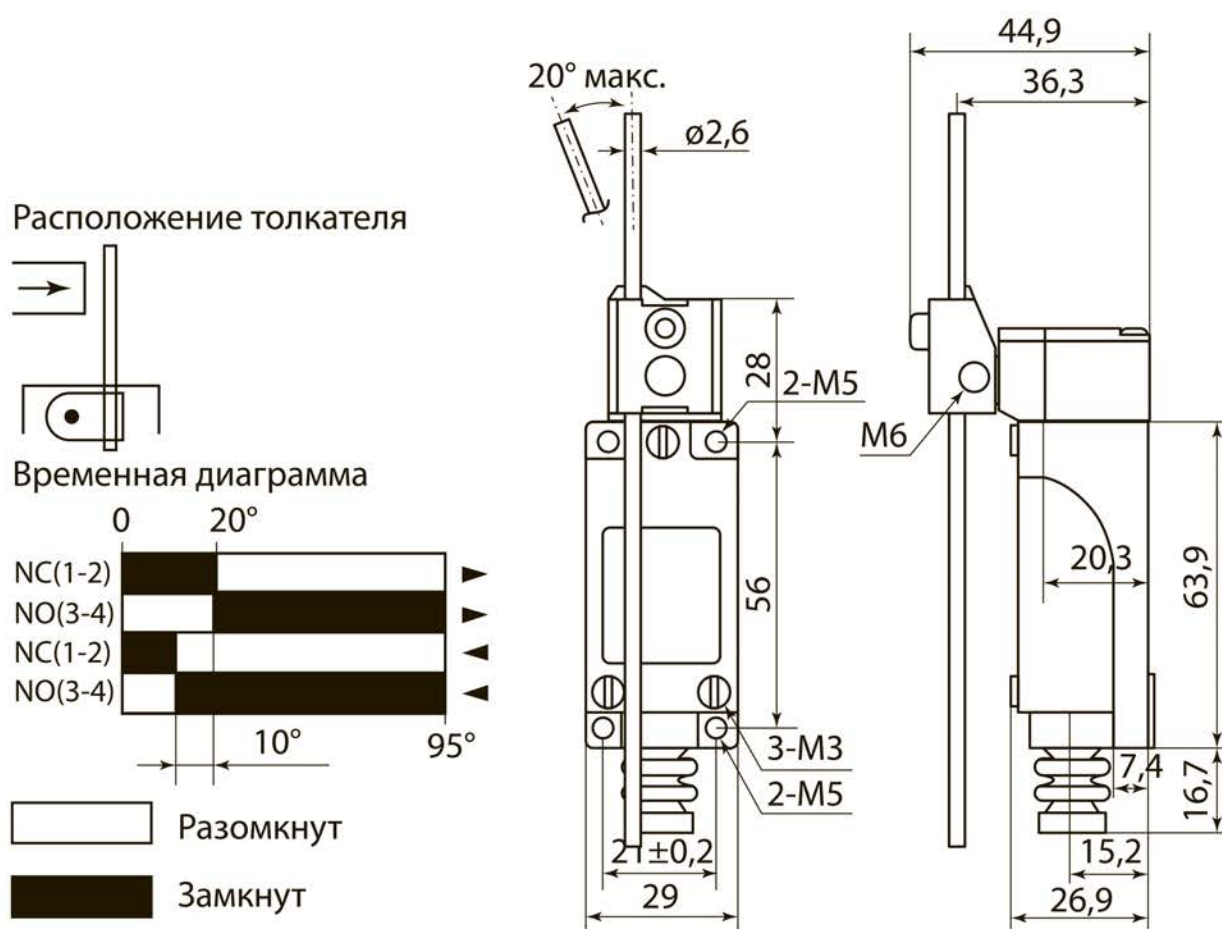
Рисунок 6. Габаритные размеры, расположение и диаграмма работы толкателя выключателя концевой ВККН-2159 М11-У2, мм
