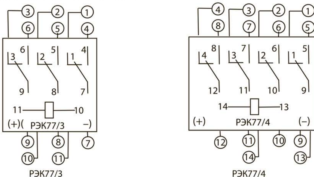
Рисунок 2. Схемы подключения
