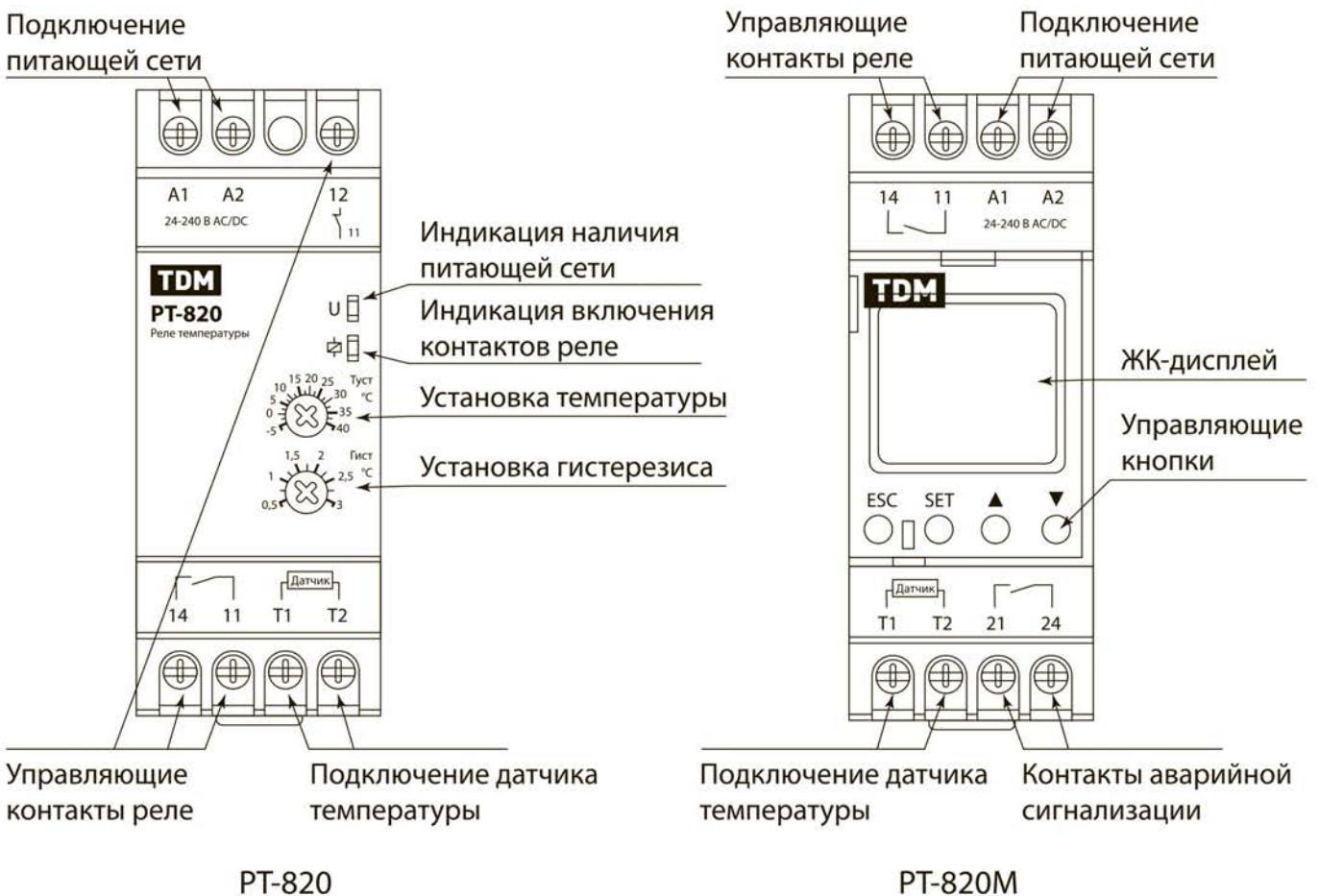
Рисунок 3. Внешний вид управляющих элементов реле
