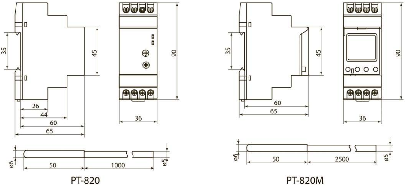
Рисунок 1. Габаритные и установочные размеры реле, мм
