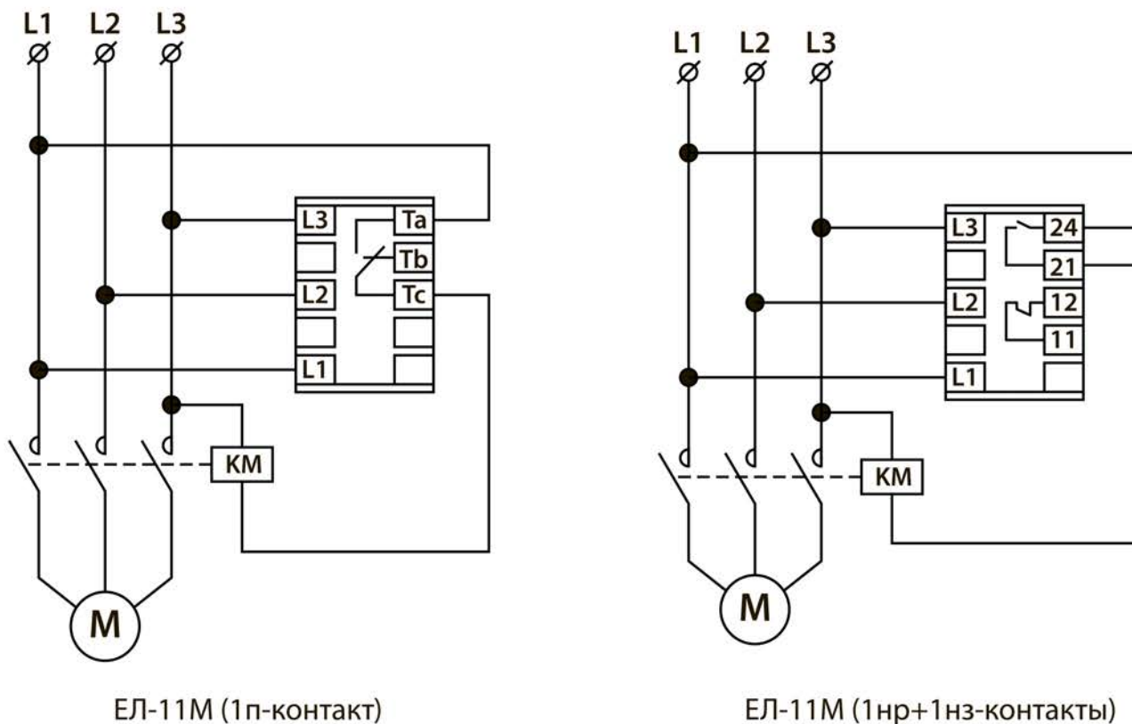
Рисунок 3. Схема подключения реле ЕЛ-11М к электрической сети
