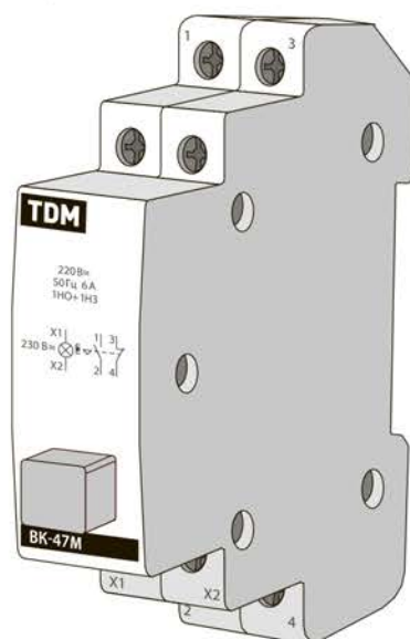
Рисунок 1. Выключатель кнопочный БК-47М
