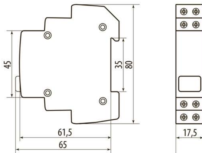
Рисунок 2. Габаритные размеры, мм
