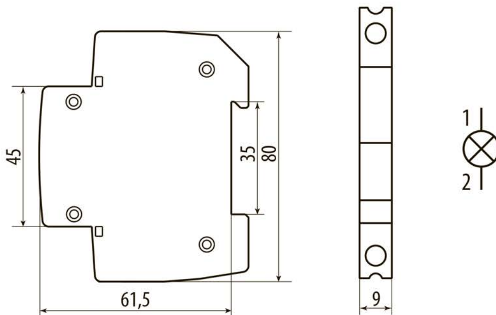
Рисунок 1. Габаритные размеры, мм
