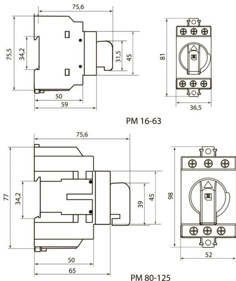
Рисунок 2. Габаритные размеры РМ (мм)
