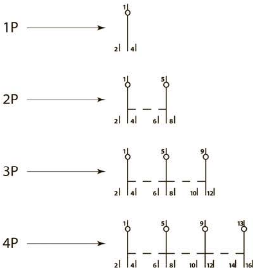
Рисунок 2. Схемы МП-125
