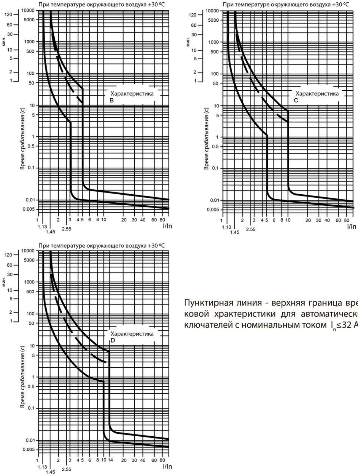
Рисунок 1. Время-токовые характеристики
