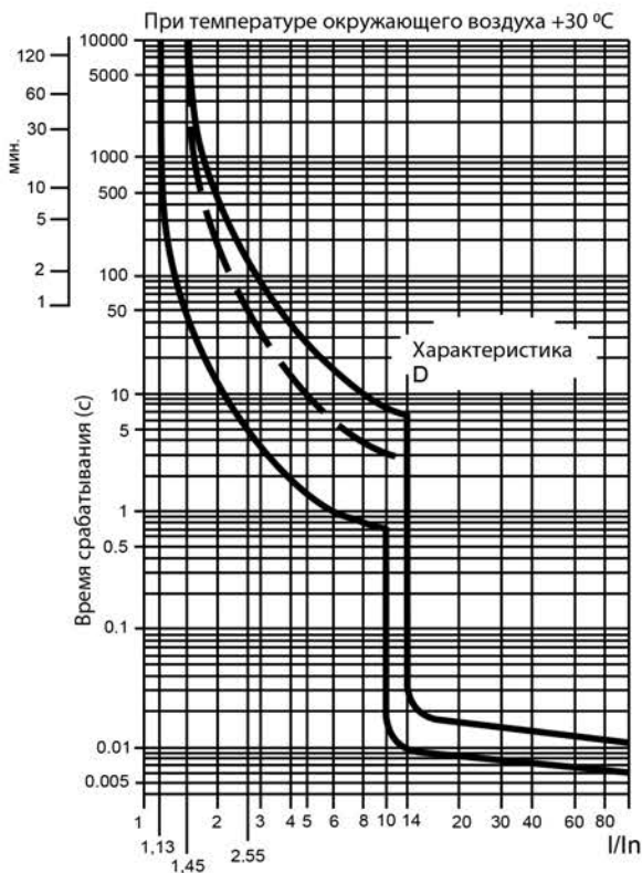
Рисунок 1. Время-токовые характеристики
